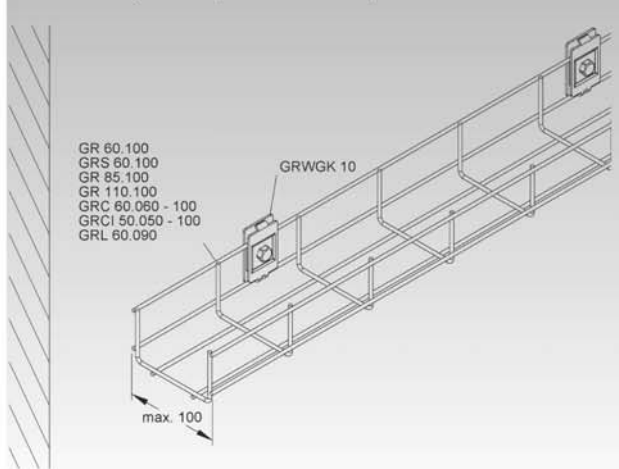
Настенное крепление проволочных лотков при помощи фиксатора GRWGK 10 (макс. ширина лотка 100 мм)
