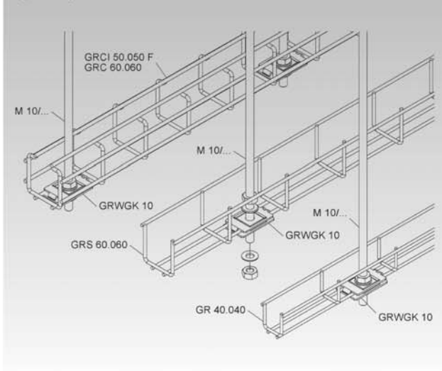
Потолочное крепление проволочных минилолков при помощи фиксатора GRWGK 10 и шпильки M10/...
