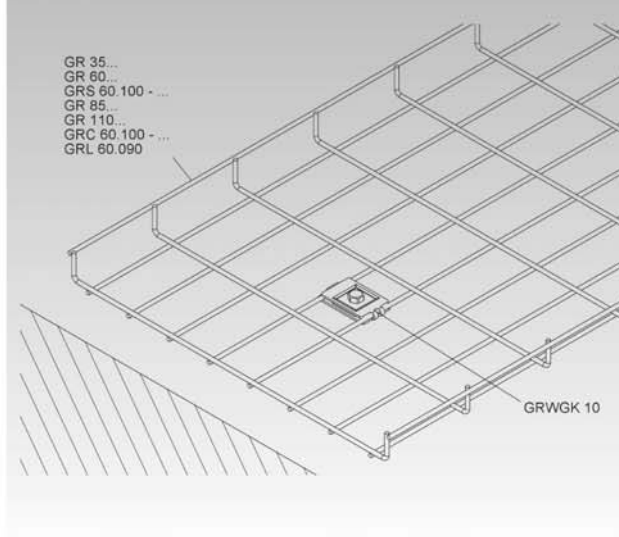
Напольное крепление проволочных лотков при помощи фиксатора GRWGK 10
