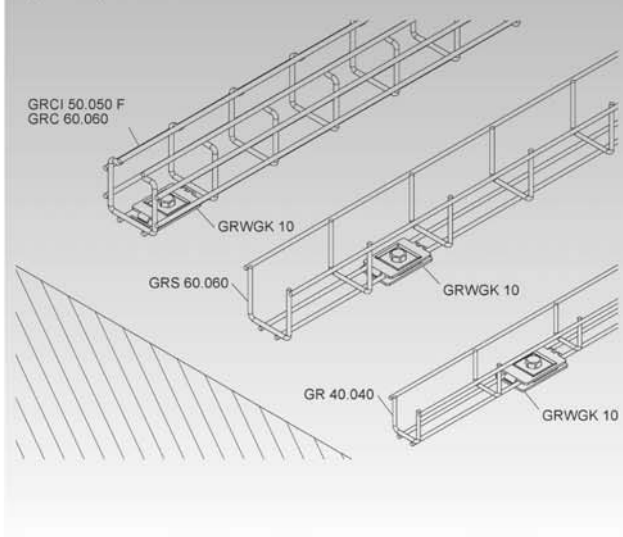
Напольное крепление проволочных минилолков при помощи фиксатора GRWGK 10
