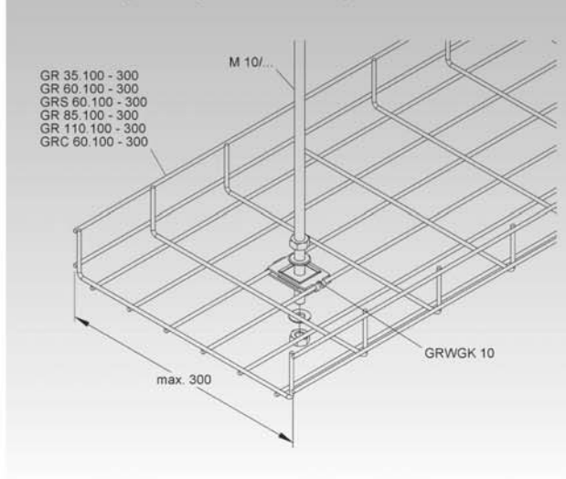
Потолочное крепление проволочных лотков при помощи фиксатора GRWGK 10 (макс. ширина лотка 300 мм) и шпильки M10/...
