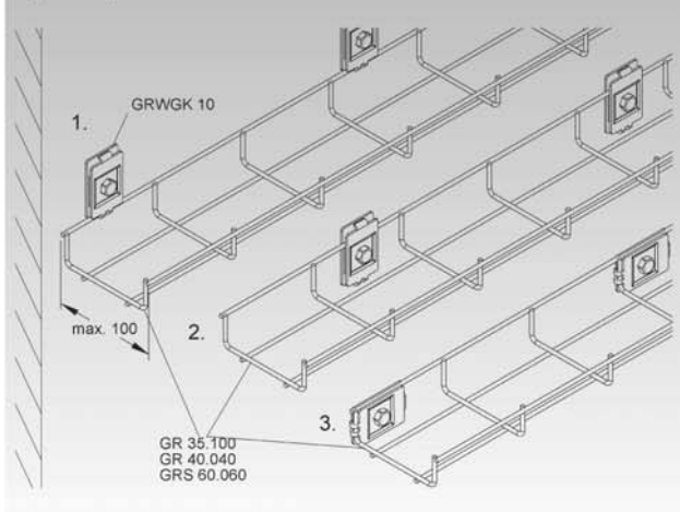
Настенное крепление проволочных минилолков при помощи фиксатора GRWGK 10
